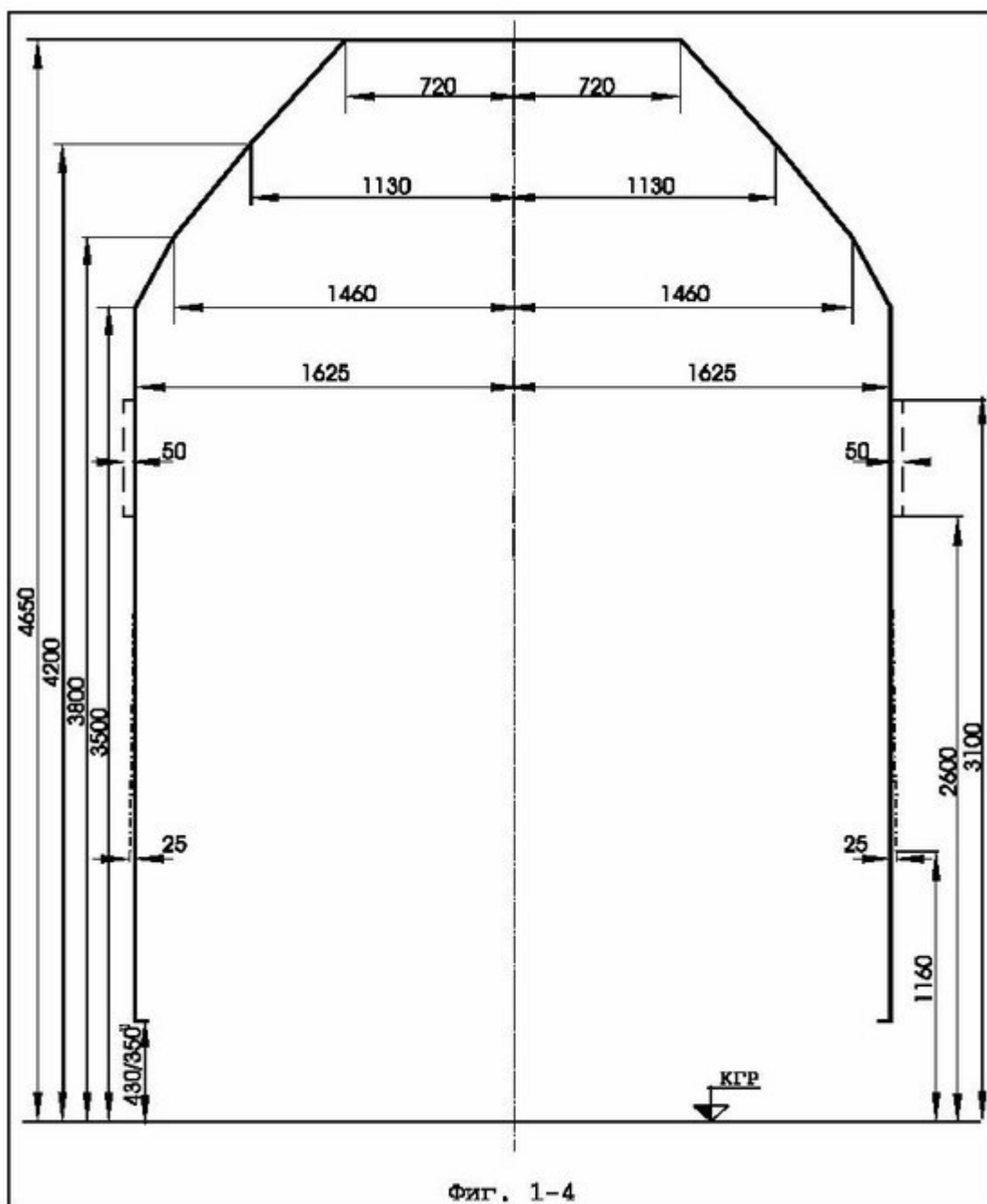
Фиг. 1-4. Статичен габарит на подвижния железопътен състав 0-ВМ (01-Т) - горна част.
