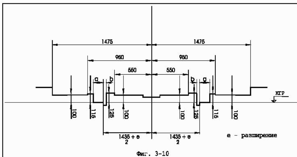
Фиг. 3-10. Строителен габарит 1-СМ 2 (долна част) за вагонозадържатели в права* (при ново строителство и преустройство)
