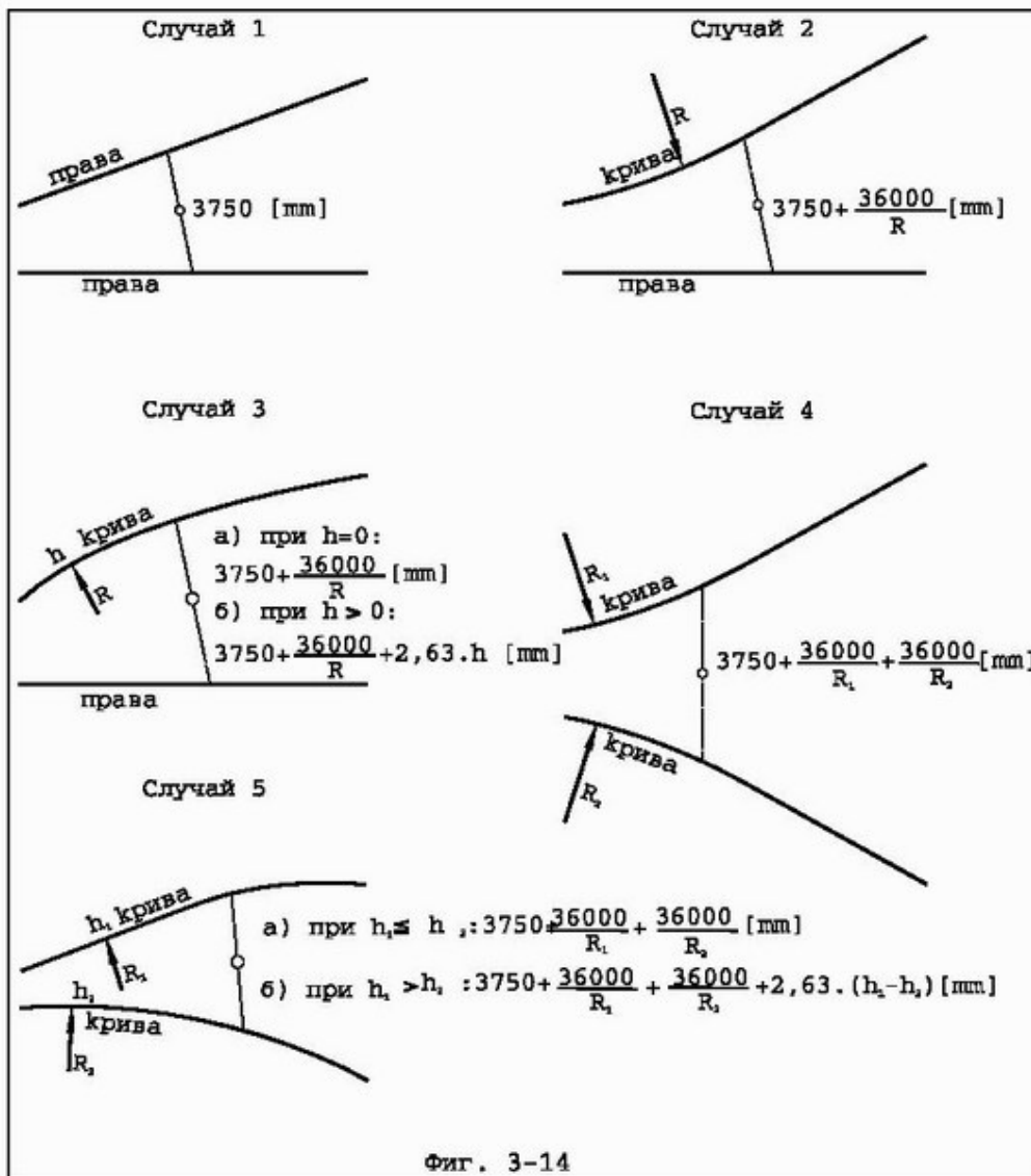
Фиг. 3-14. Разстояние между осите на съседни коловози при дистанционните знаци за железопътни линии със стандартно междурелсие 1435 mm.
