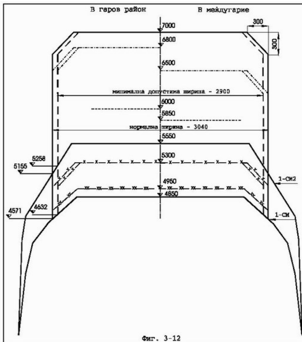
Фиг. 3-12. Строителен габарит на надстройката за електрифицирани жп линии с горен проводник за променливо напрежение 25 kV, 50 Hz в права*
