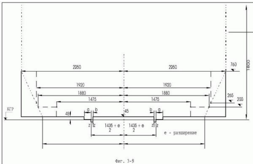
Фиг. 3-9. Строителен габарит 1-СМ 2 за стоманени жп мостове система "Трог" без баластова призма и жп естакади на разтоварища за жп линии в права*
