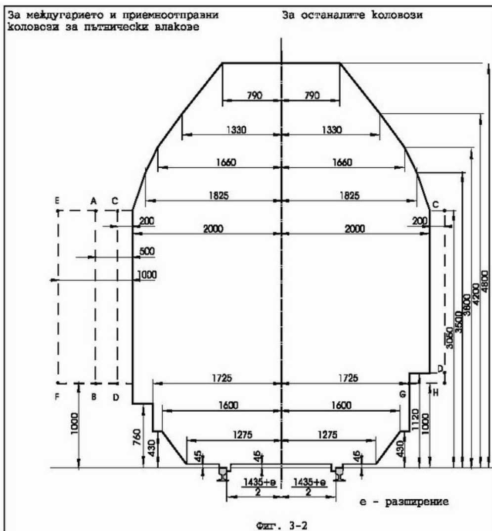
Фиг. 3-2. Строителен габарит 0-СМ за прави и криви с R \geq 250 m.
