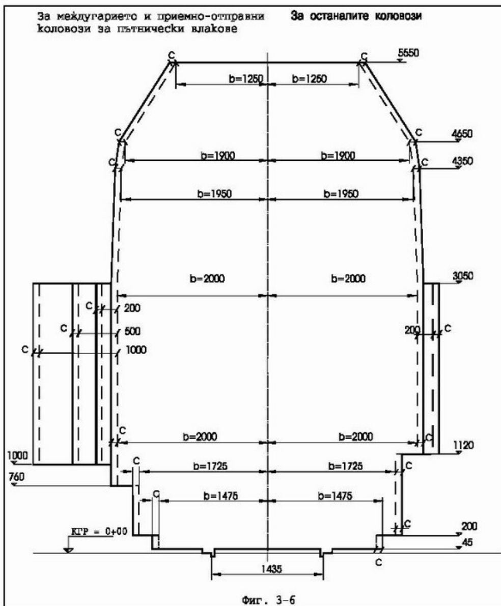
Фиг. 3-6. Строителен габарит 1-СМ 2 за жп линии в крива без надвишение
