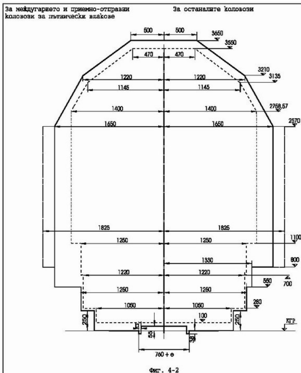
Фиг. 4-2. Строителен габарит за 760 mm в права*
